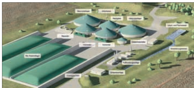
Luftbild und 3D-Modell der Biogasanlage Weißenborn-Lüderode
